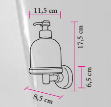
art. 6810110 PORTA SAPONE LIQUIDO DA MURO Fusioni di bronzo, finiture cromo/oro 24k
