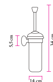
art. 6810078/B PORTASCOPINO DA PARETE Fusioni di bronzo, finitura palladio, inserti in vetro blu, interno in vetro WALL BRUSH HOLDER Die-cast bronze, palladium finish, blue glass interior, glass inserts
