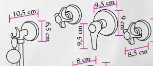
art. 6810094 GRUPPO VASCA ESTERNO Fusioni di bronzo, dor. oro 24K Pezzi per il montaggio inclusi OUTSIDE BATHTUB UNIT Die-cast bronze, 24K gold plated Assembly parts included
