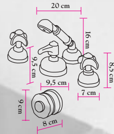
art. 6810040 GRUPPO BORDO VASCA QUATTRO FORI CON DOCCIA ESTRAIBILE E COLONNA EROGATORE AL TROPPO PIENO Fusioni di bronzo, finiture cromo/oro 24k (Pezzi per il montaggio inclusi)
