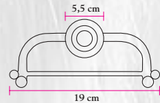
art. 6810037 PORTAROTOLO Fusioni di bronzo, finitura palladio PAPER ROLL HOLDER Die-cast bronze, palladium finish
